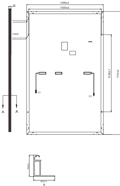
Dimensions du module PV
